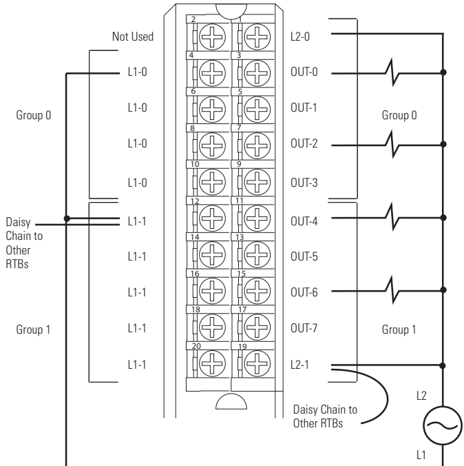
1756-0A8E
