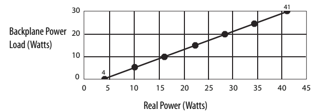
1756-PB30XT (DC)
