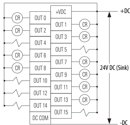
1769-0V16
