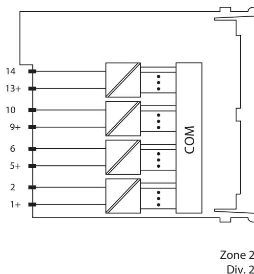
I/O module
