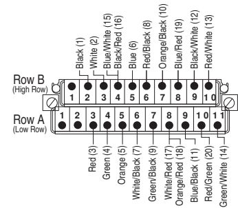
1492-CAB0F64
