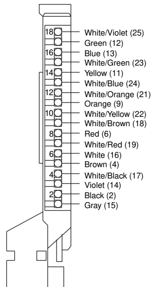
1492-ACABLE___J
