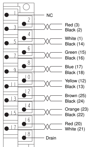
1492-ACABLE___C
