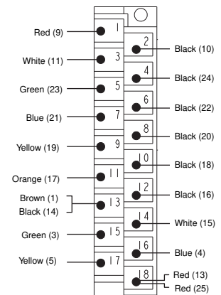
1492-ACABLE___P*
