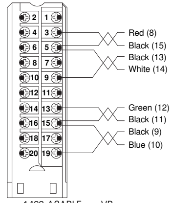
1492-ACABLE___VB
