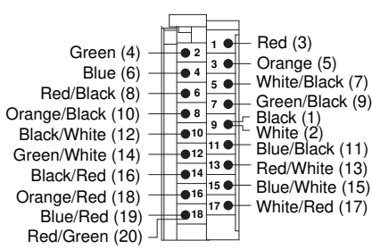
1492-CAB1B69
