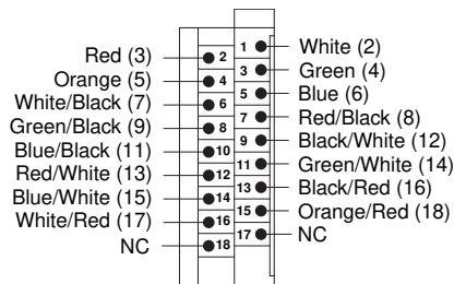
1492-CAB1D69
