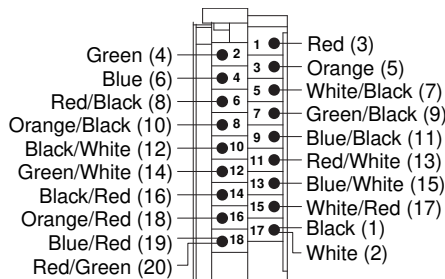
1492-CAB1A69
