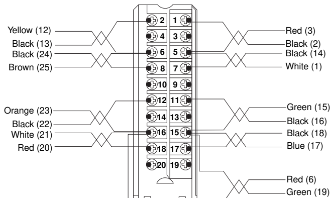
1492-ACABLE___WA
