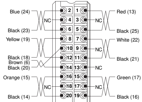
1492-ACABLE___Y
