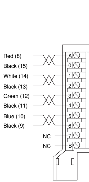
1492-ACABLE___G
