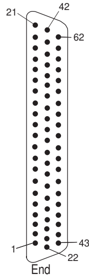
1492-CAB0H94 ③
