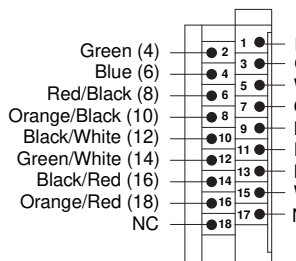
1492-CAB1F69
