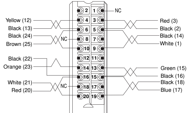
1492-ACABLE___WB
