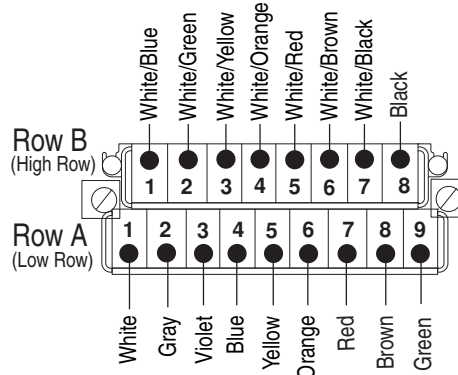
1492-CAB0RTN32L
