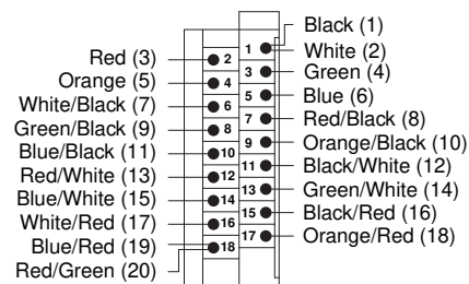
1492-CAB1E69
