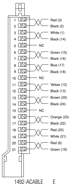
1492-ACABLE___E
