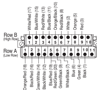
1492-CAB1B64
