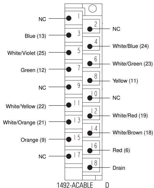
1492-ACABLE___D
