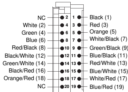
1492-CABLE 1V
