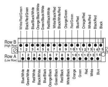
1492-CAB0U64
