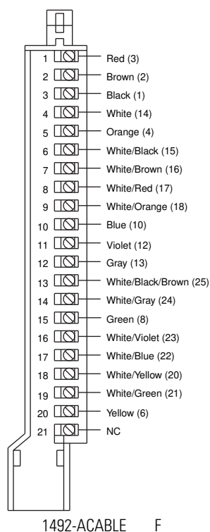
1492-ACABLE___F
