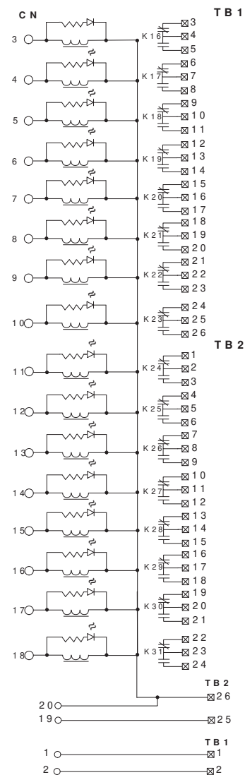
1492-XIM2024-16R
