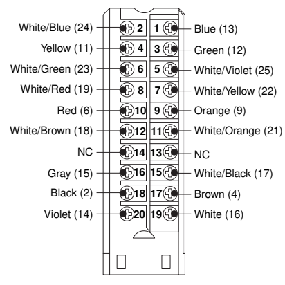
1492-ACABLE___Z
