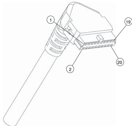
20-Conductor Cable
