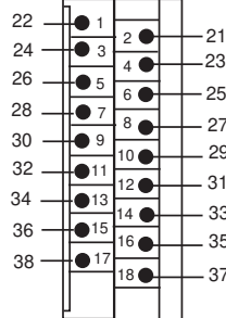
1492-CAB0RTN32L
