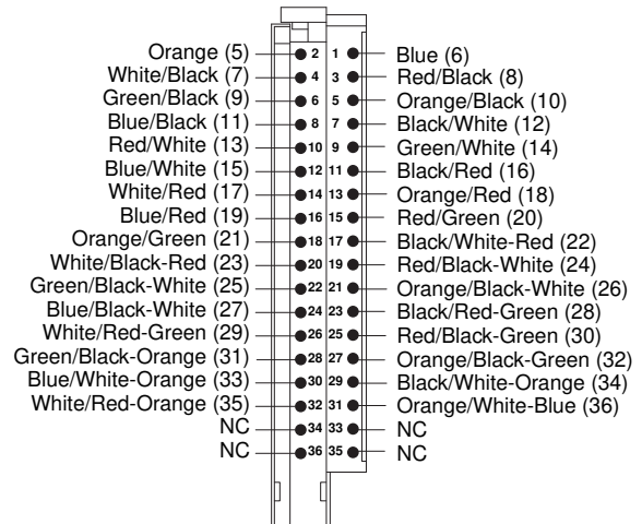
1492-CABLE 1Y
