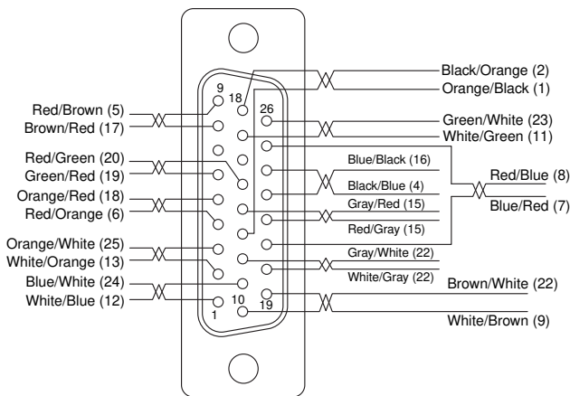
1492-ACABLE___Q
