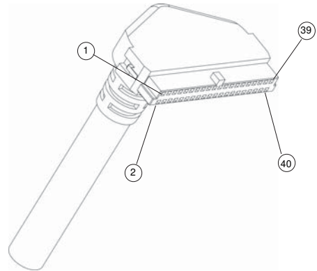
40-Conductor Cable
