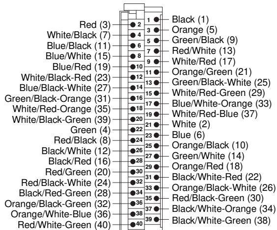
1492-CABLE 1R
