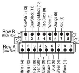
1492-CAB1A64
