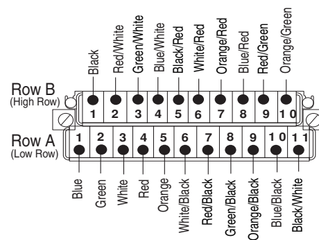
1492-CAB0U64
