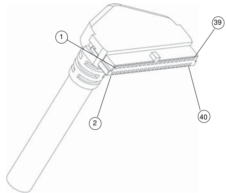
40-Conductor Cable
