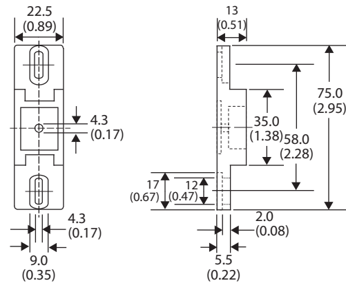
Cat. No. 199-FSA...
