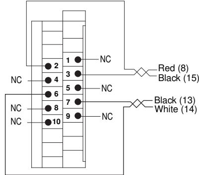
1492-ACAB__AB69
