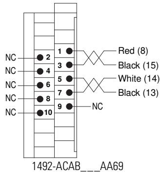
1492-ACAB__AA69
