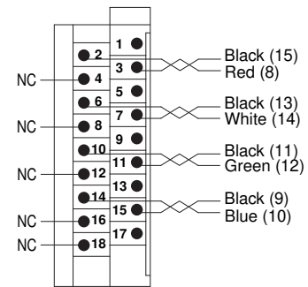
1492-ACAB__BD69
