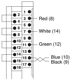
1492-ACAB__BB69
