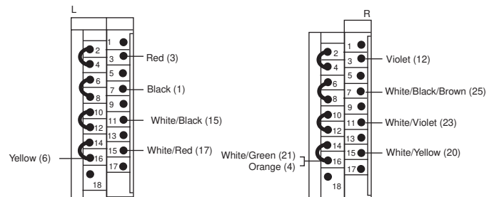
1492-ACAB__EB69 ①
