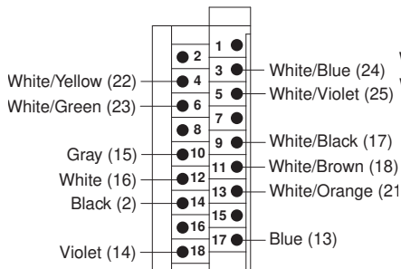
1492-ACAB__CA69
