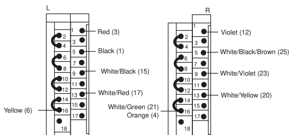
1492-ACAB__EA69 ①
