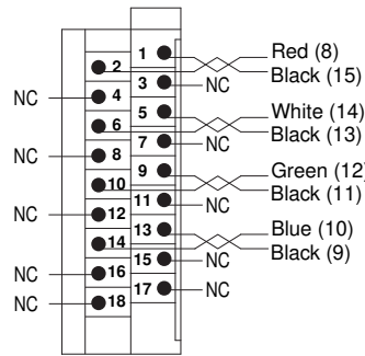
1492-ACAB__BC69
