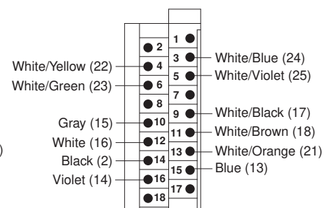
1492-ACAB__CC69
